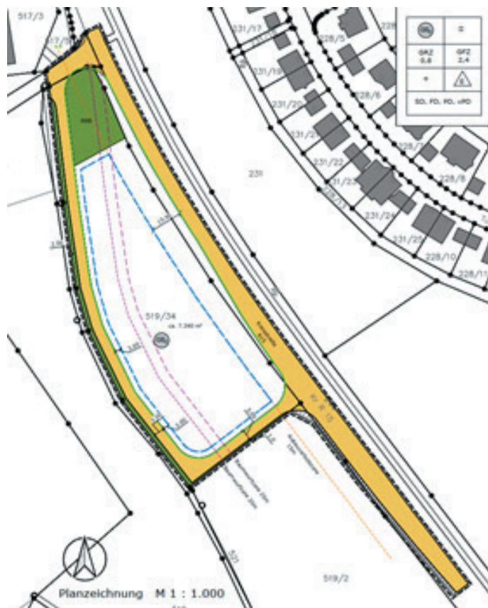
Auszug Bebauungsplan; verkleinerte Darstellung ohne Maßstab; Bearbeitung Markt Lappersdorf
